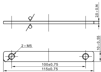
固定板 Fixed plate
