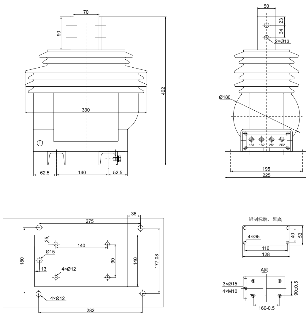
LZZBW-10 电流互感器外形图及安装尺寸
