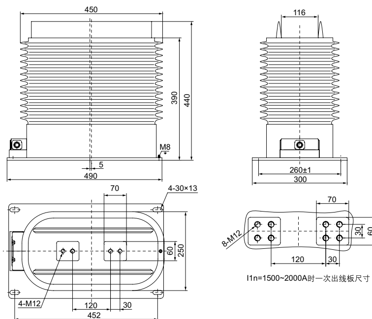
LZZBJ9-35 型电流互感器三绕组外形图及安装尺寸
