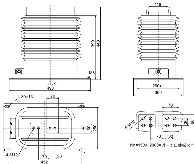
LZZBJ9-35 型电流互感器两绕组外形图及安装尺寸
