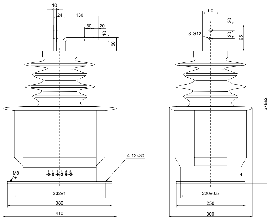
LZZB7-35 电流互感器外形图及安装尺寸
