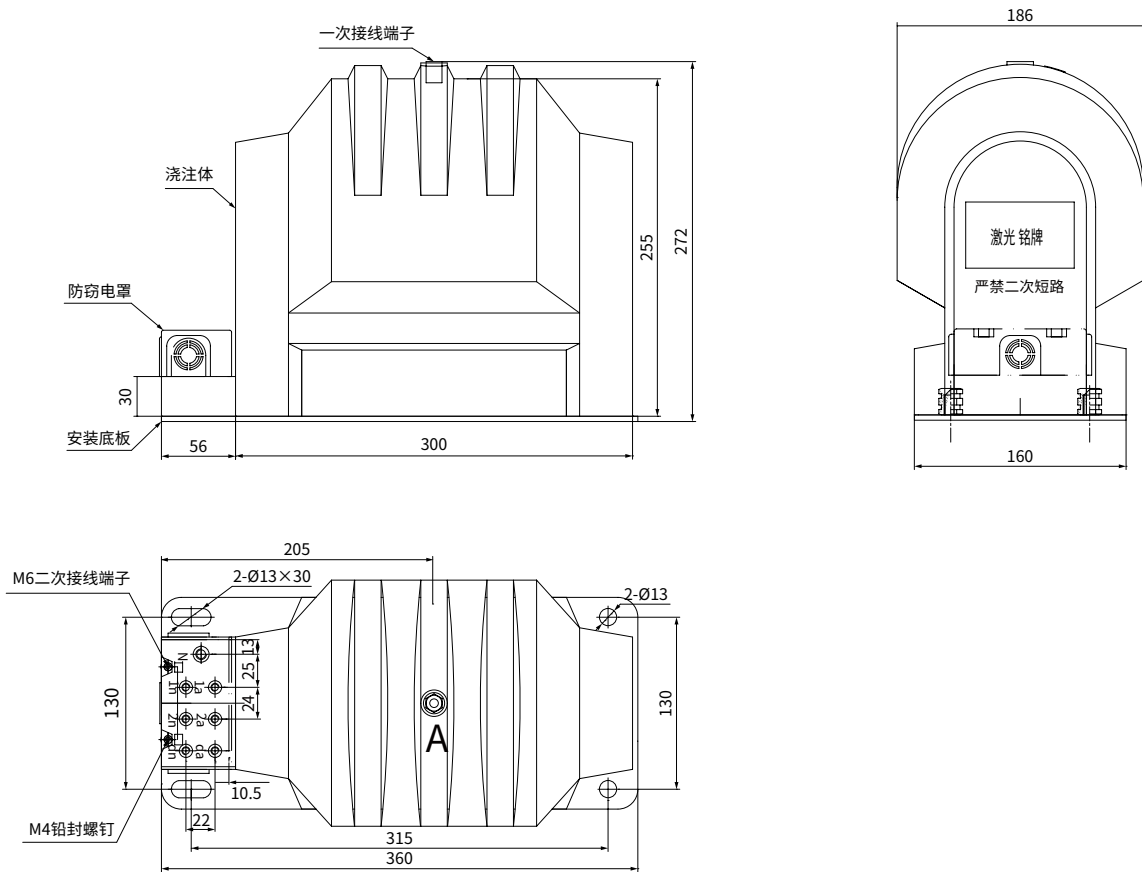
JDZX9-3、6、10D 电压互感器外形图及安装尺寸 JDZX9-3、6、10D Voltage transformer outline drawing and installation dimensions
