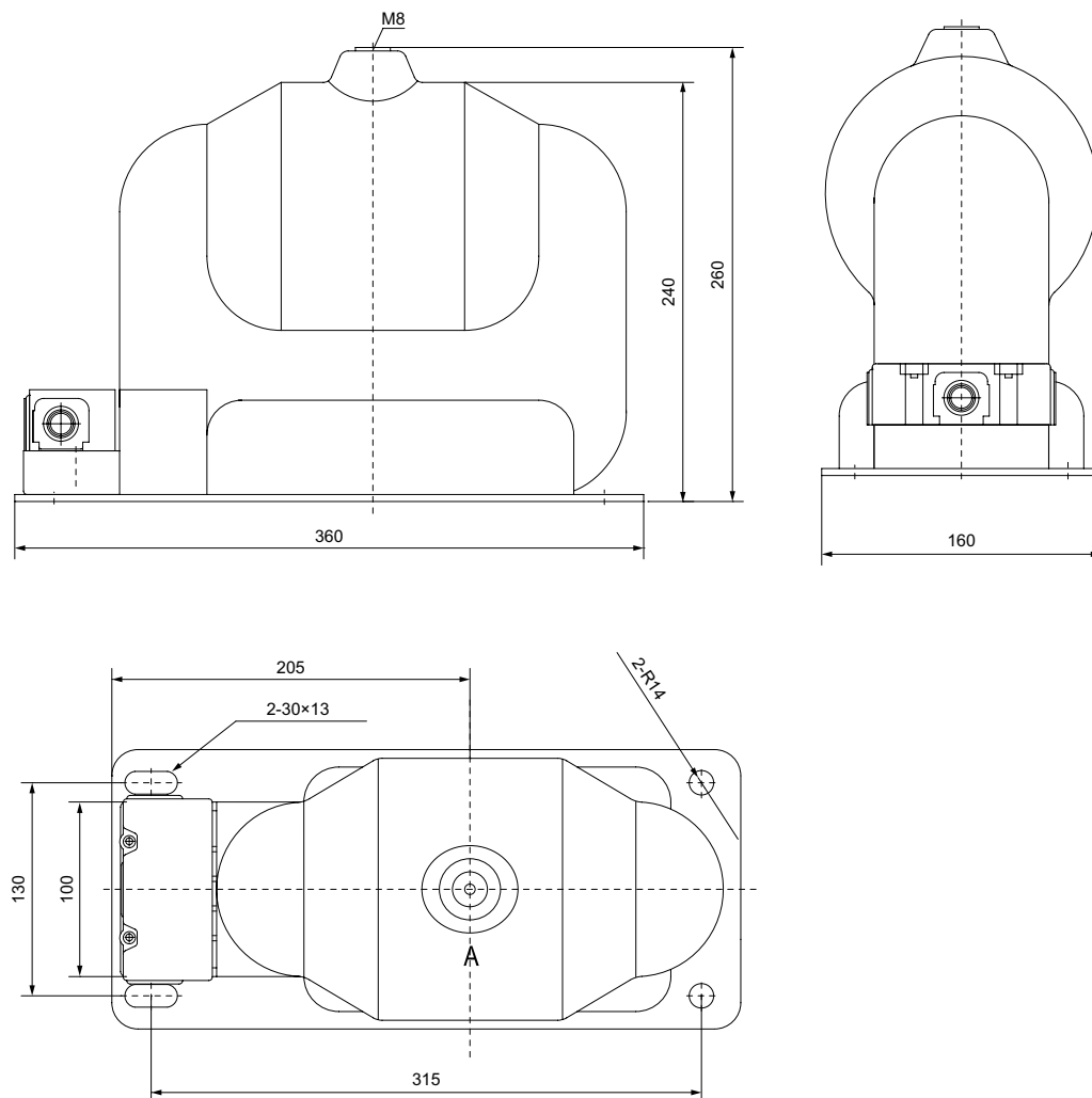
JDZX9-3、6、10 电压互感器外形图及安装尺寸
