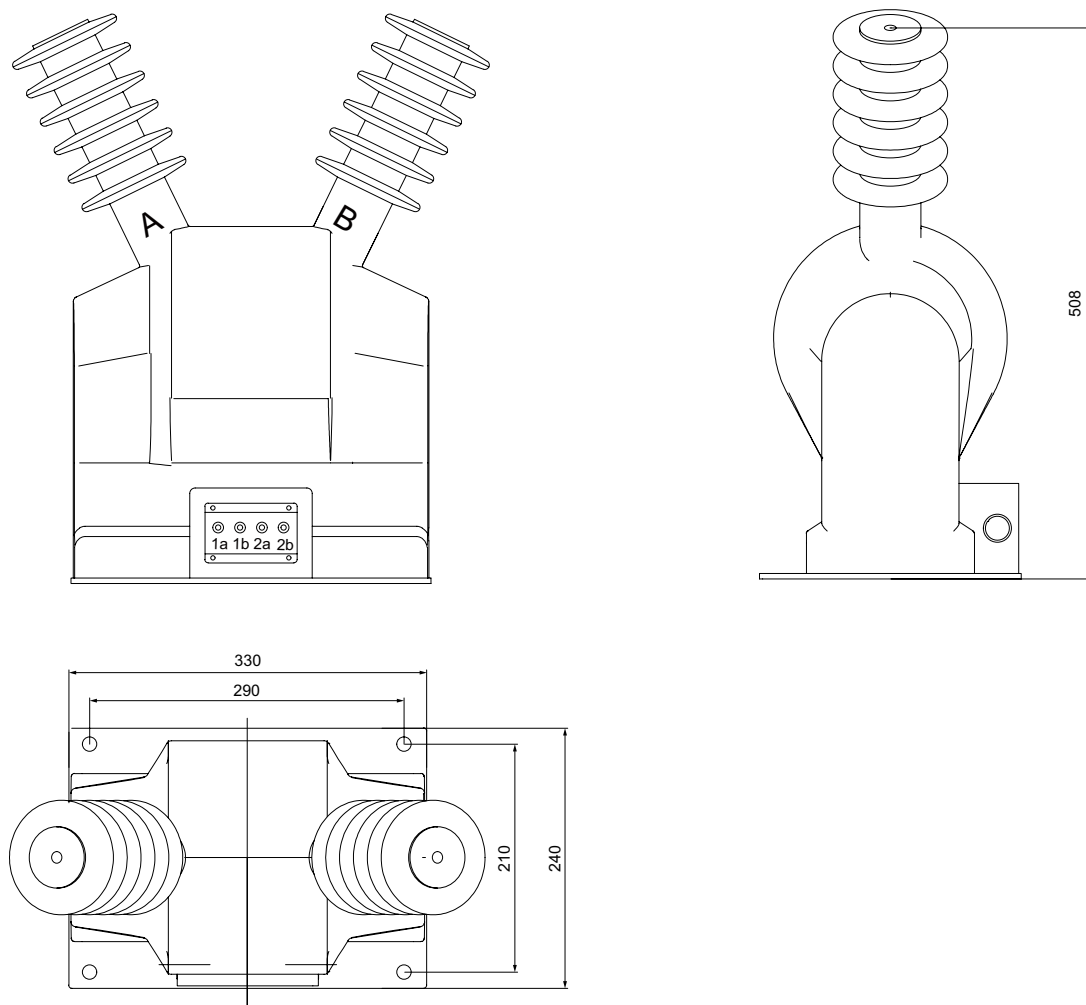
JDZXW-15 电压互感器外形及安装尺寸图
