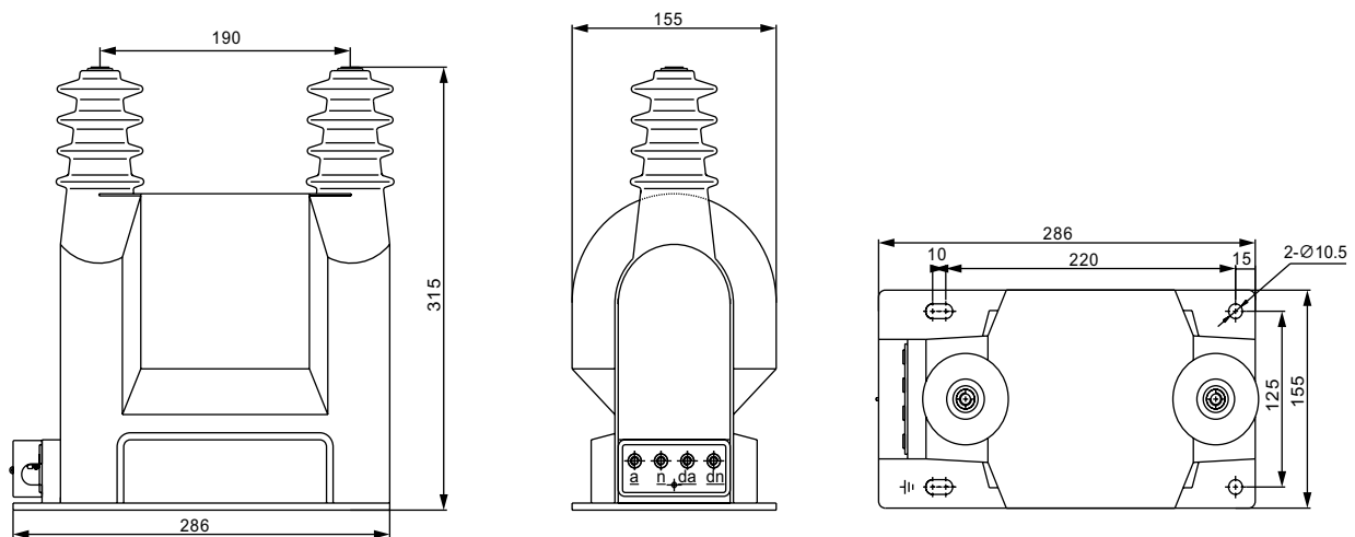
JDZJ(18)-3、6、10 电压互感器外形图及安装尺寸图
