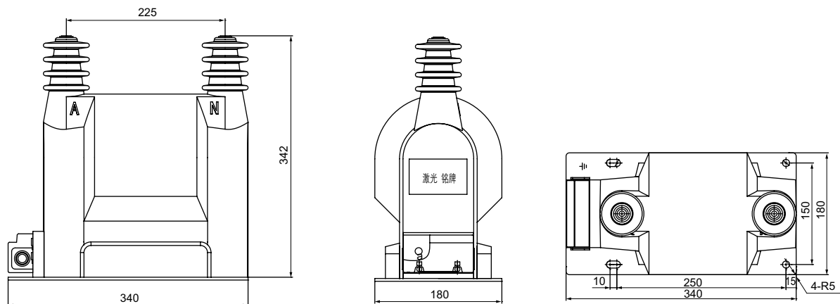
JDZJ(18)-3、6、10 电压互感器 (0.2/0.5/6P) 外形图及安装尺寸图
