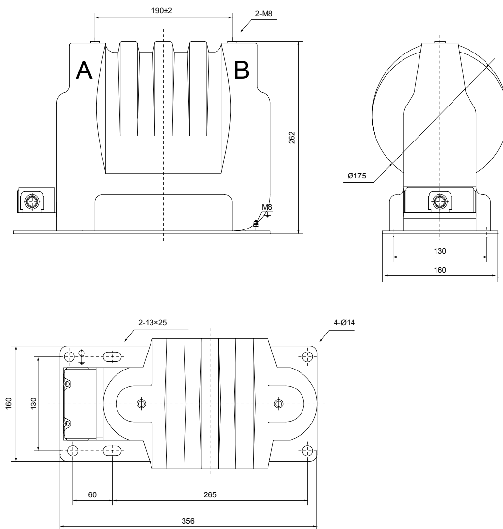
JDZ9-3、6、10 电压互感器外形图及安装尺寸 JDZ9-3、6、10 Voltage transformer outline drawing and installation dimensions
