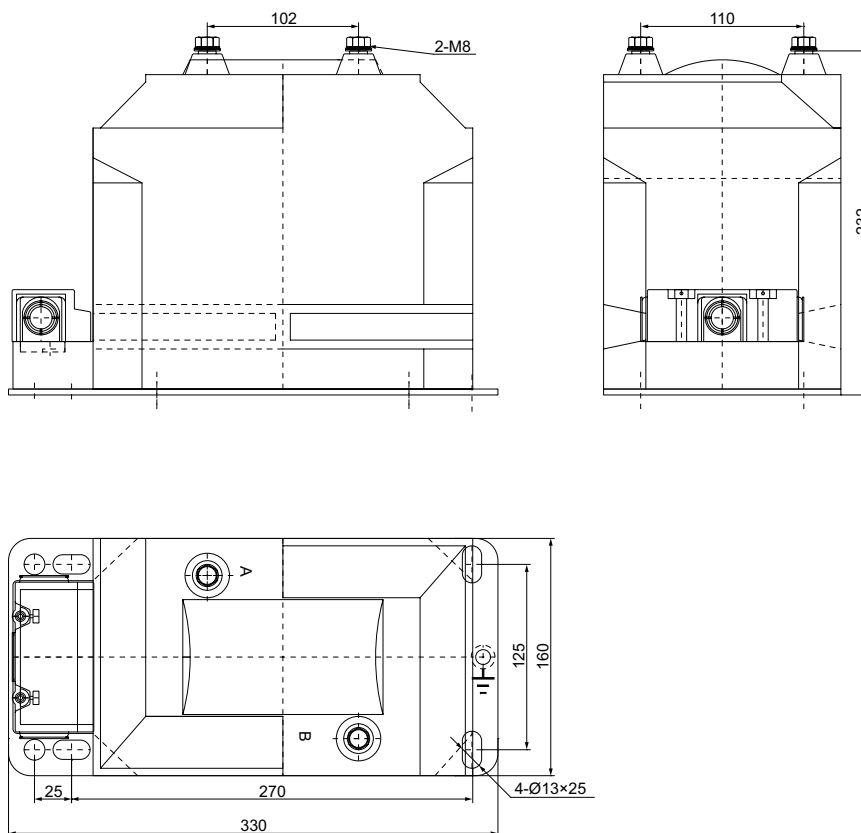
JDZ10-3、6、10 电压互感器外形图及安装尺寸 JDZ10-3、6、10 Voltage transformer outline drawing and installation dimensions
