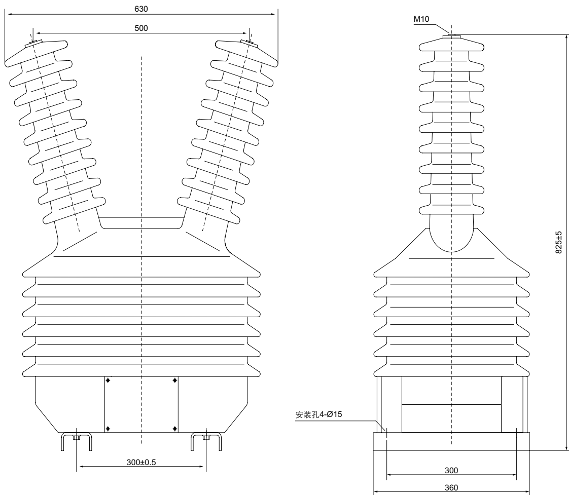
JDZ(X)W-35 型电压互感器外形图及安装尺寸
