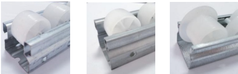
TAPER TYPE 鼓轮 FLAT TYPE 平轮 FLANGE TYPE 挡边轮
