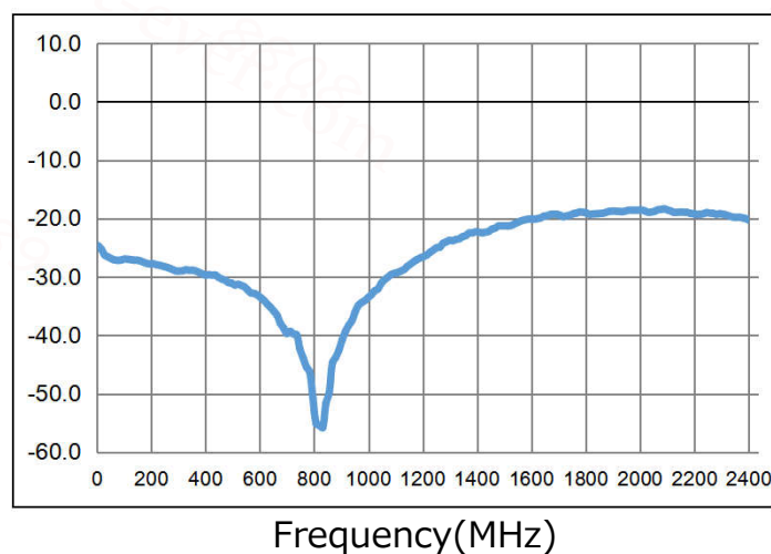
Input Return Loss(Pin6)
