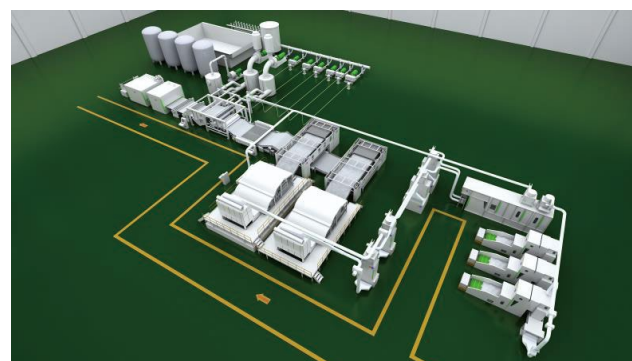
■ 水刺非织造布生产线 Spunlaced Nonwovens Production Line
