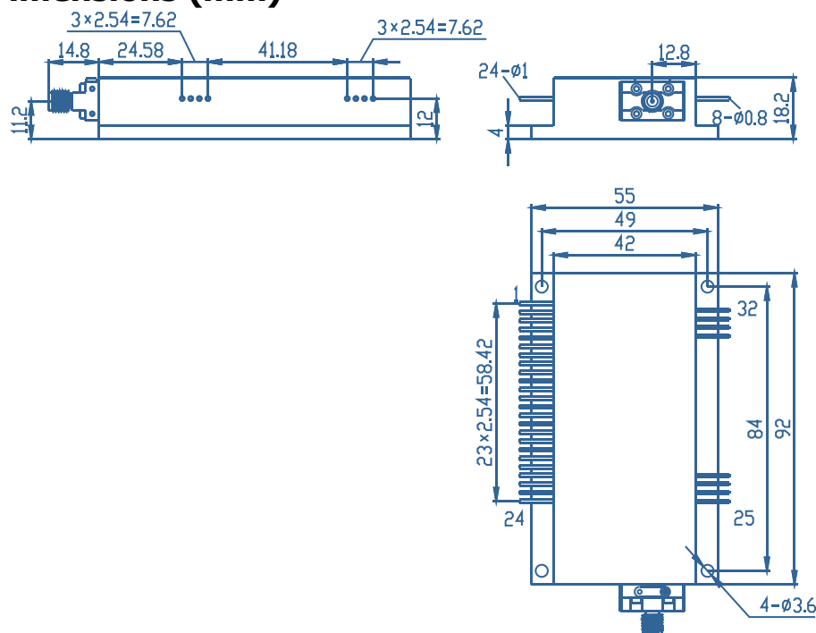
引脚功能分配 Pin-Out Assignment
