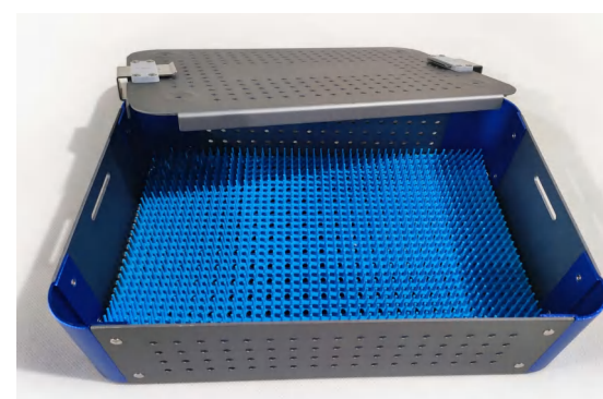
LHJ-251602 250*160*25 mm
