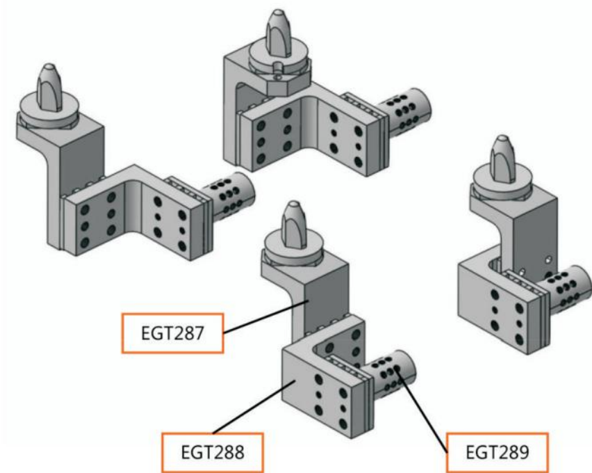
3.3 定位销单元
