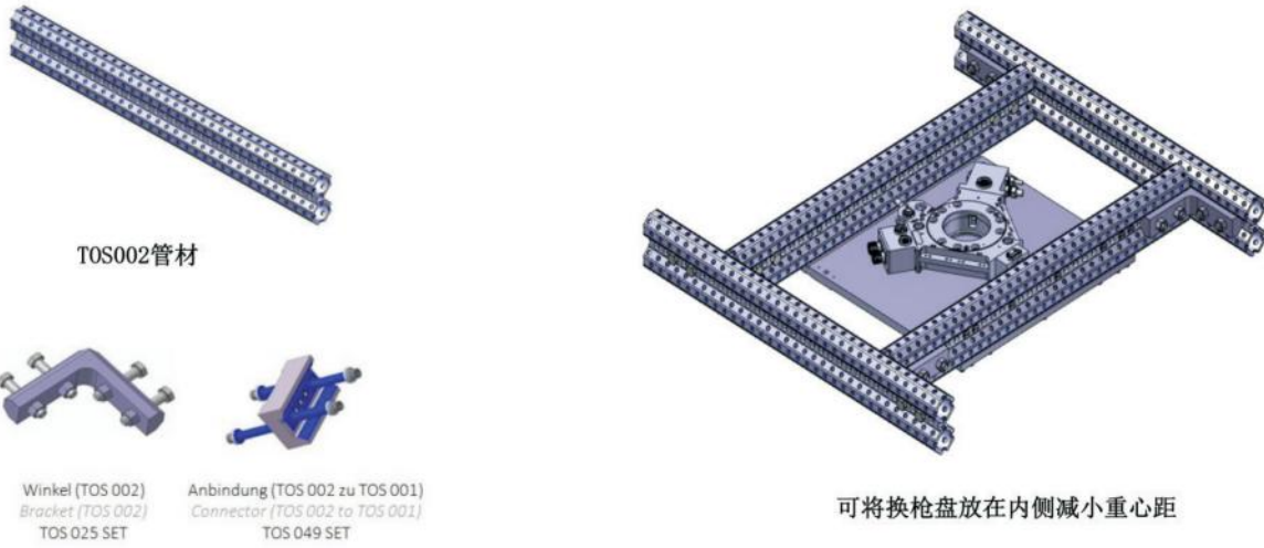
TOS002框架连接件
