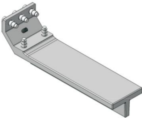
尺寸: 236mm x 88mm x 116mm
