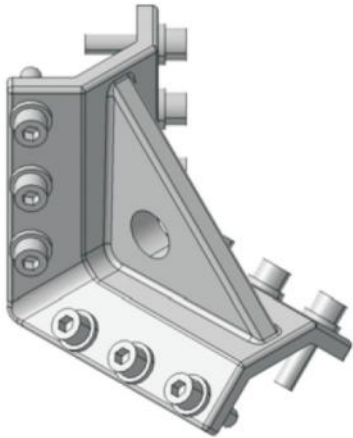
尺寸: 111mm x 111mm x 79mm
