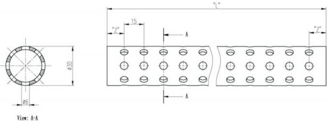
EGT006 最大长度: 1000mm
