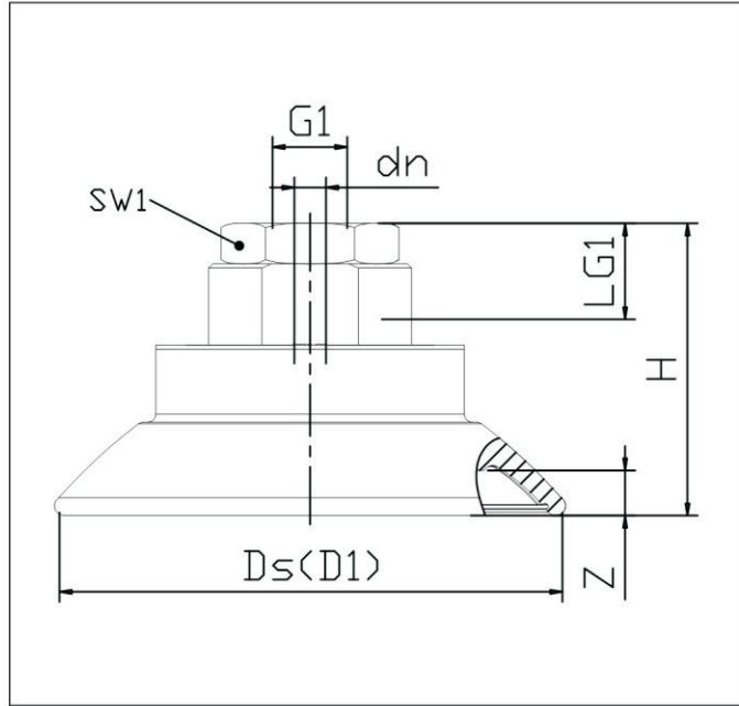
MAF 30 至 100 IG
