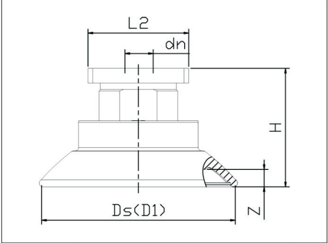
MAF 30 至 100 RA (矩形适配器)
