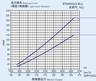
锅炉燃烧器功率(kW) Burner Output (kW)
