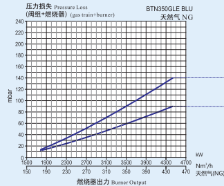
锅炉燃烧器功率(kW) Burner Output (kW)
