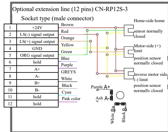
YK-HL8030U-SSN-2-815 Wiring Diagram
