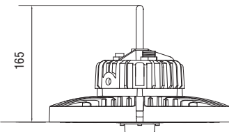
JD-HB032B-150W
