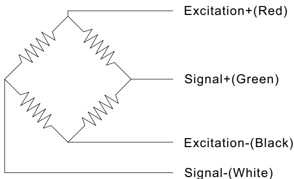
Wiring Code
