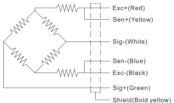
Wiring Code@Clockwise
