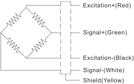
Wiring Code
