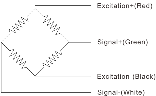
Wiring Code
