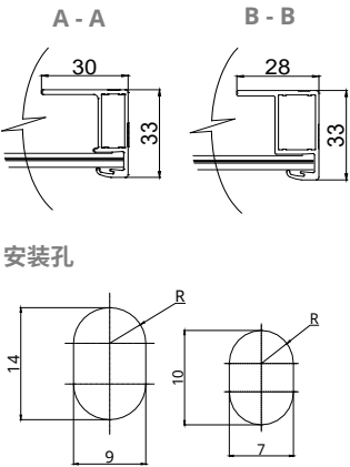
边框横截面
