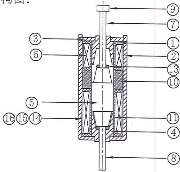
产品结构图:
