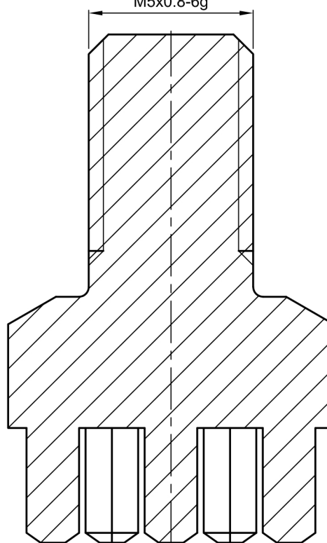
SECTION A-A
