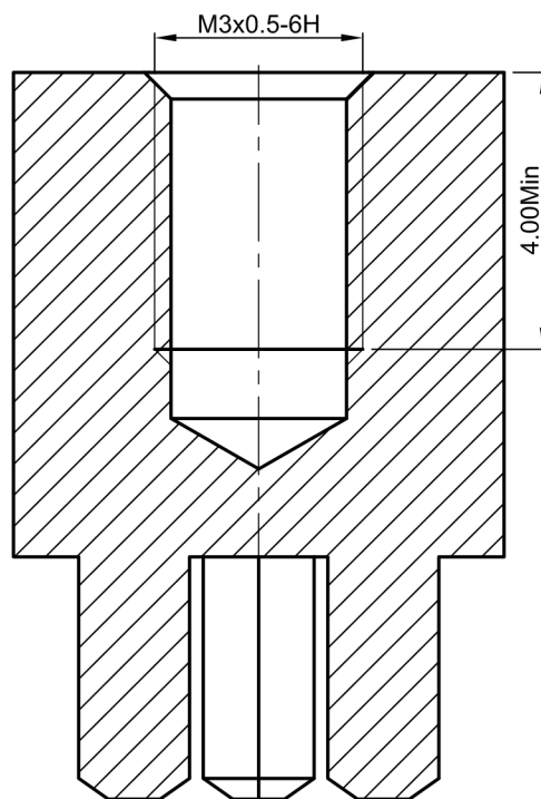
SECTION A-A
