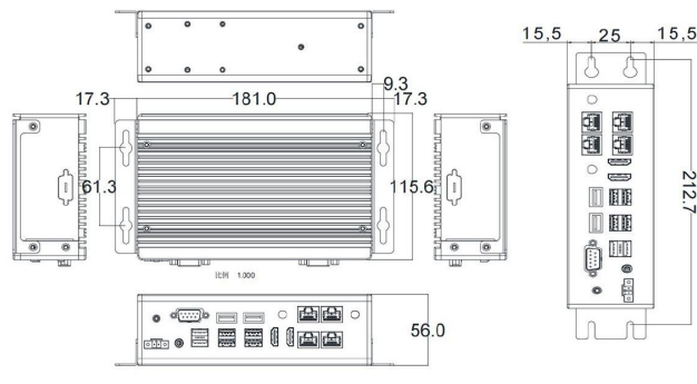
■ 尺寸图
