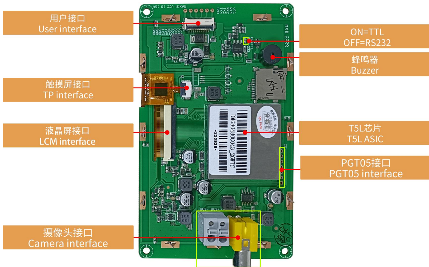
硬件接口图
