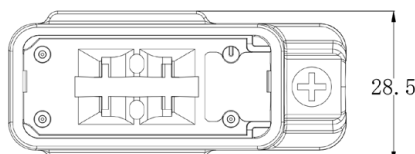
Structure 2: y=2(28.5mm)
