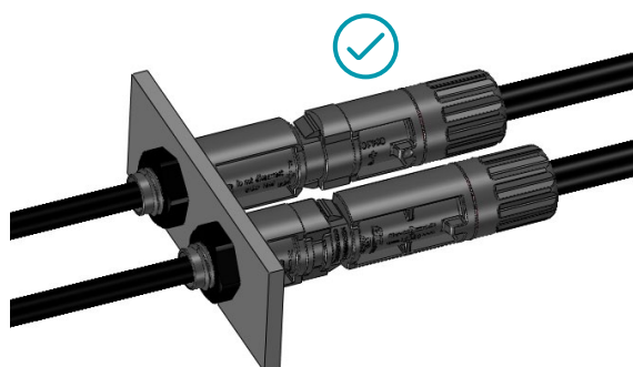
正确的接合示意图 in right place
