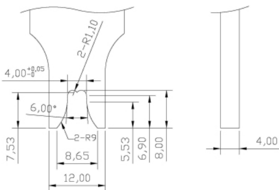
上刀尺寸 Tool Size(Up)
