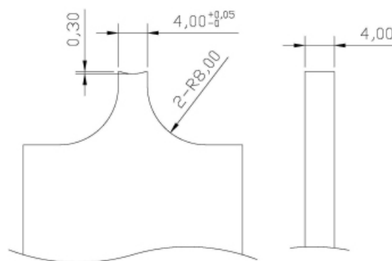
下刀尺寸 Tool Size(Down)
